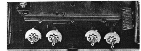
Abb. 5 Schalterachsen ein- und ausbauen
