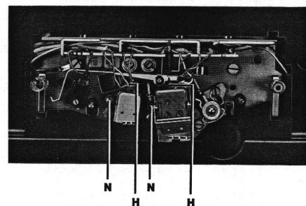
Kopfjustage
