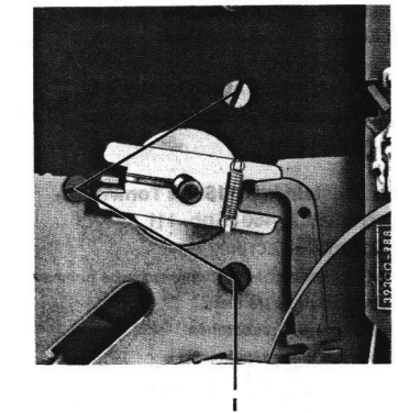
Abb. 9 Wickelmotor
