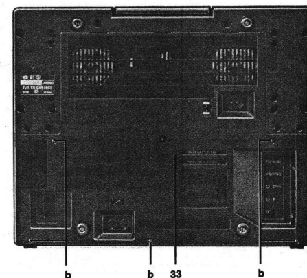
Abb. 2 Rückansicht
