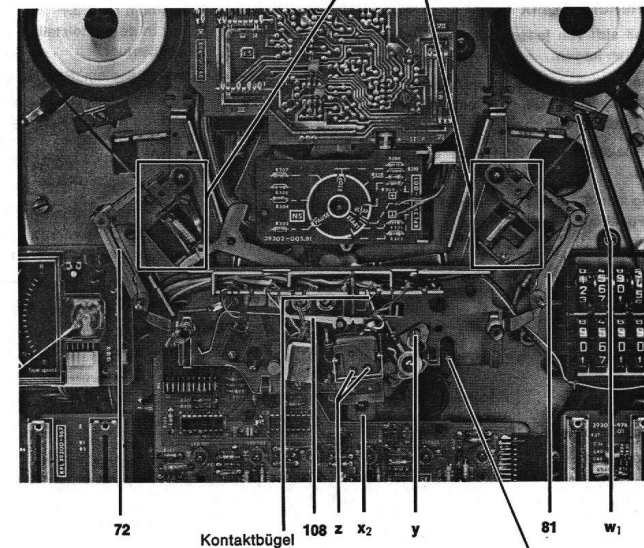
Abb. 13 Justage
