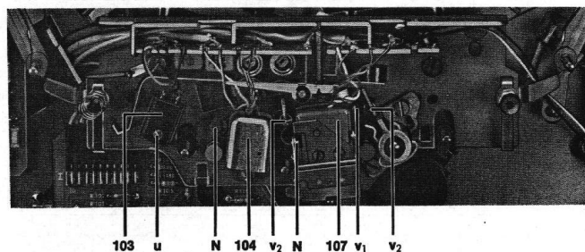
Abb. 12 Kopfwechsel
