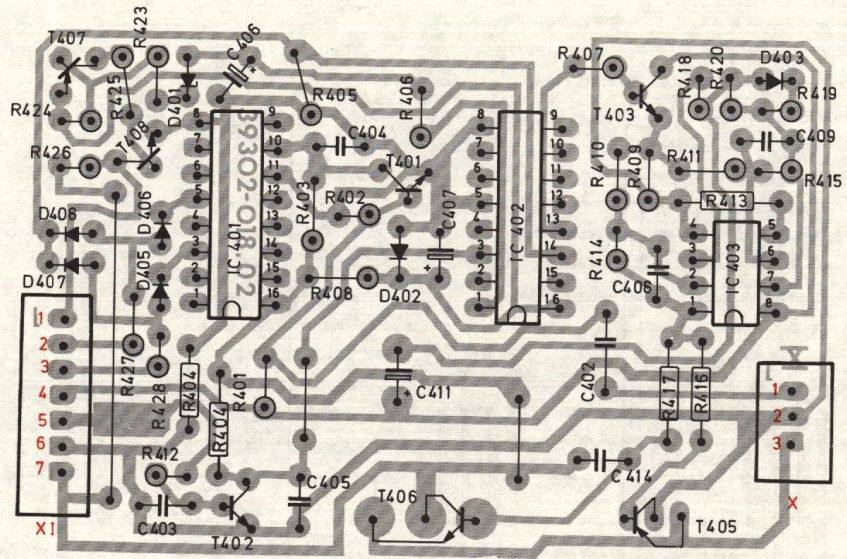
Tonwellen - Motorregelung
