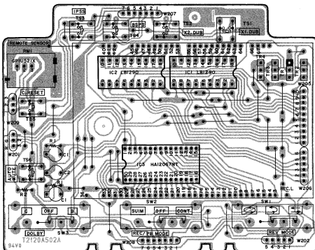
DISPLAY PCB T2120A502A
