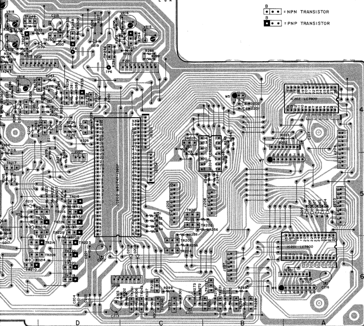
DISPLAY PCB T2120A502A
