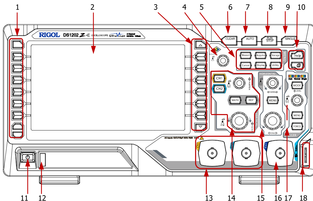
Bild 1-9 Bedienfeld Übersicht
