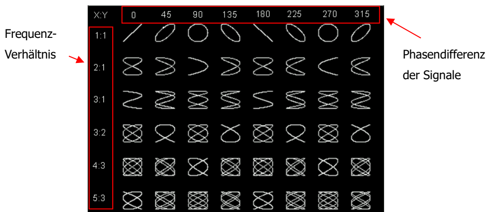
Abbildung 6-2 eingebaute Lissajous-Schemas
