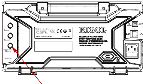
BNC-Buchse "Triggenerausgang"
