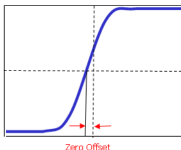
Bild 2-1 Zero Offset
