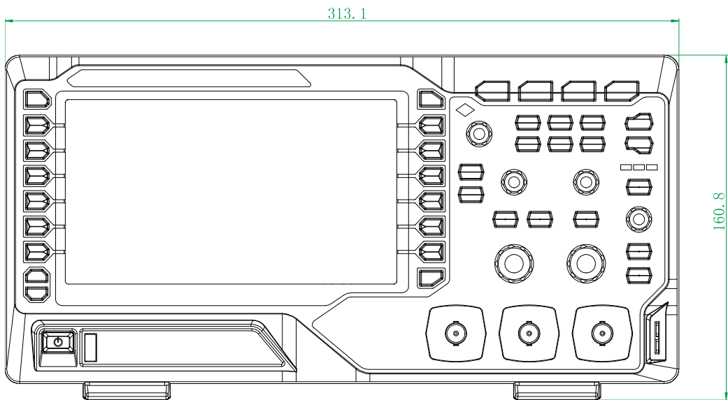
Bild 1-1 Frontansicht
