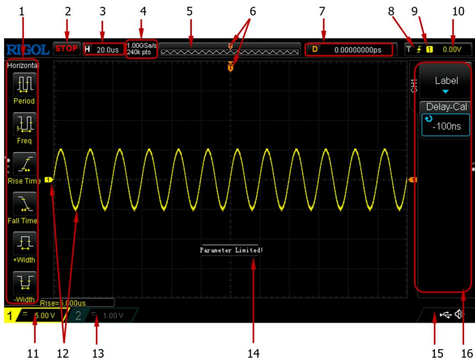
Bild 11 Benutzeroberfläche
