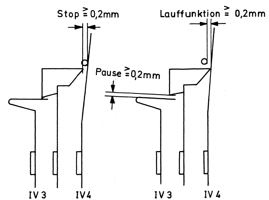
Kontaktfedersatz S 1 (Laufwerkunterseite)
